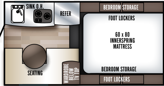
1/2 TON 5'6" OR 6'6" BED
